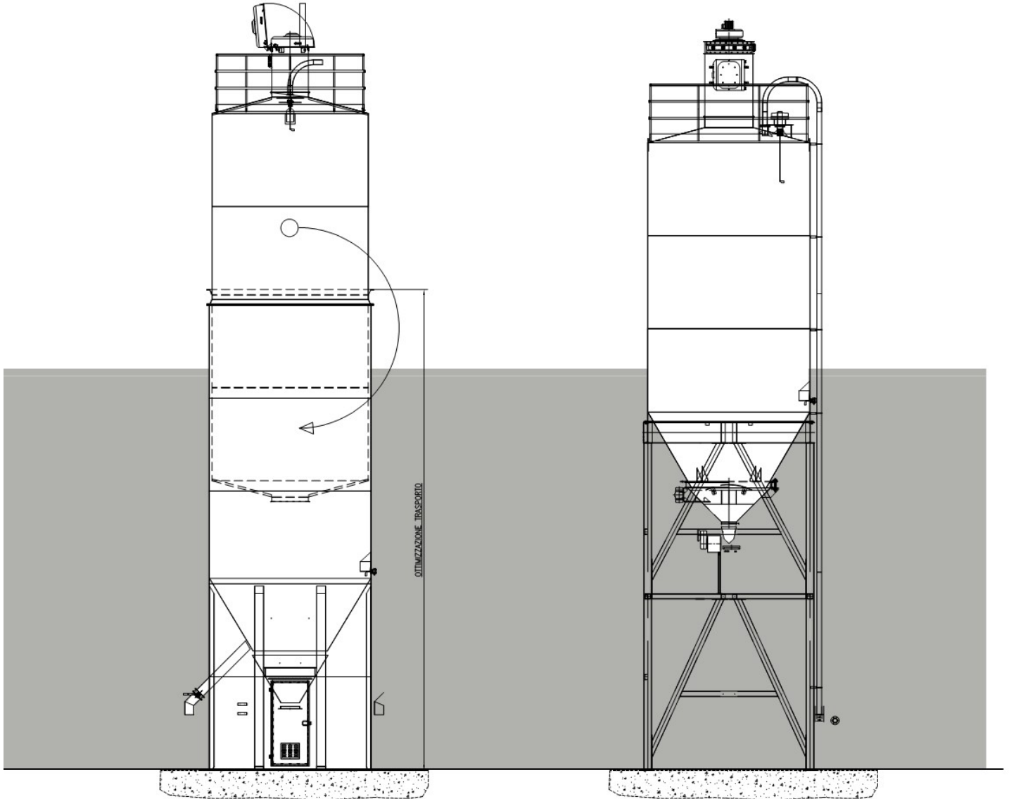
SILOS ESTENSIBILE PER OTTIMIZZARE TRASPORTO SU NAVE EXTENSIBLE SILOS TO OPTIMIZE SHIP TRANSPORT
